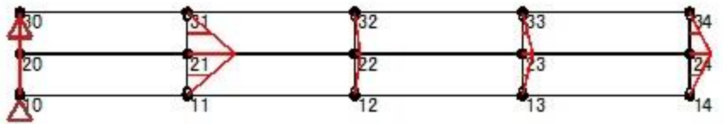
軸力図
